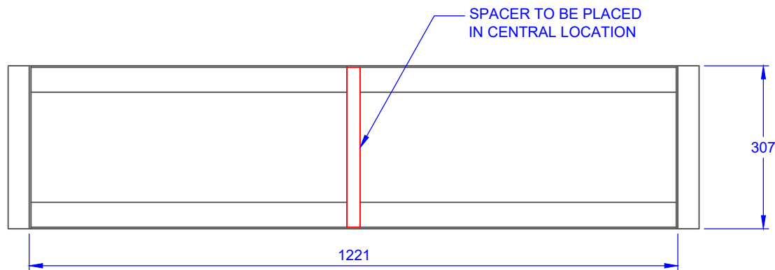
TOP VIEW TLJ05 TROUGH & SPACER BAR N.T.S.
