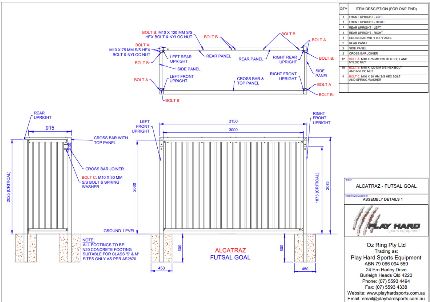
Fig: Alcatraz Assembly
